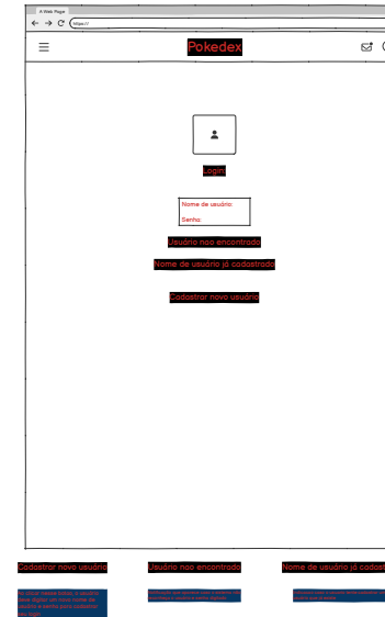
Wireframe login
