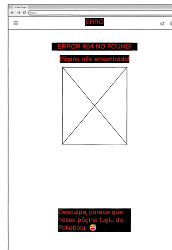
Wireframe erro 404
