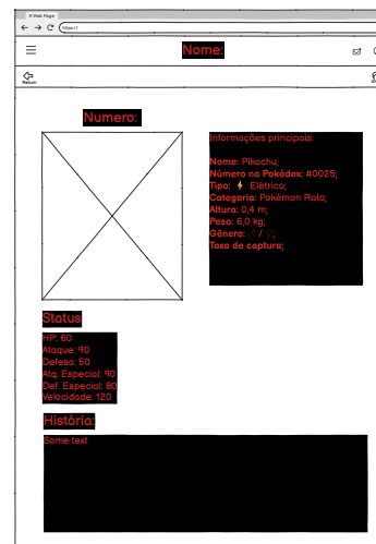
Wireframe pokemon
