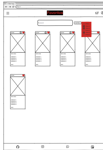
Wireframe favoritos
